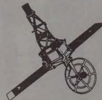
MARINER II (VENUS 1962)
